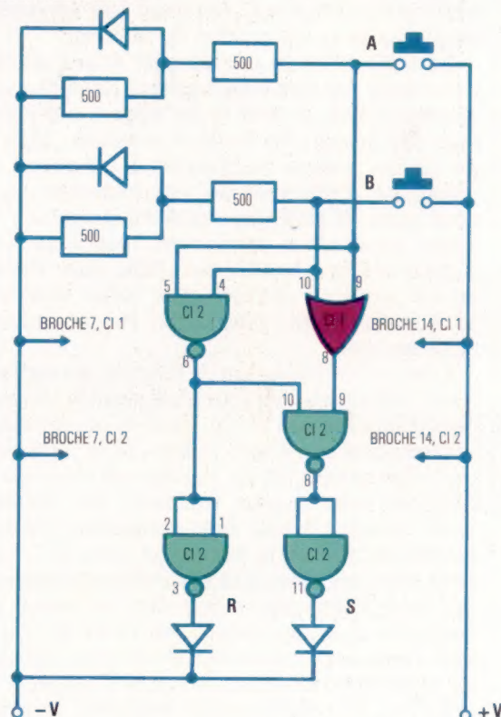
CIRCUIT ÉLECTRONIQUE
